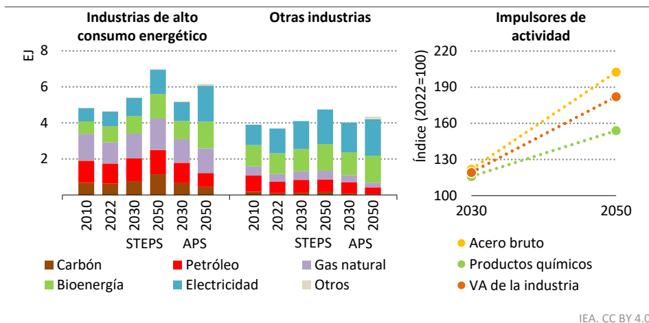
Figura 2 ▶ Consumo de combustible en la industria por tipo y escenario en ALC
