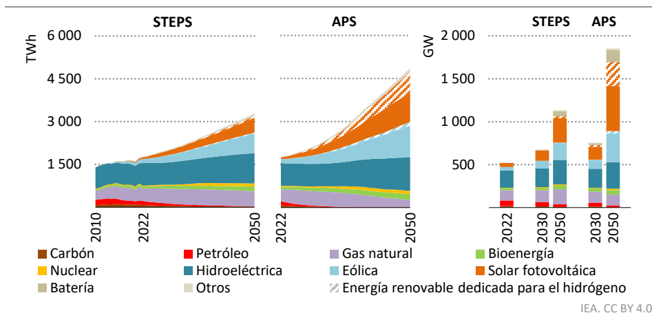
Figura 5 ▷ Generación y capacidad de electricidad por combustible en ALC
