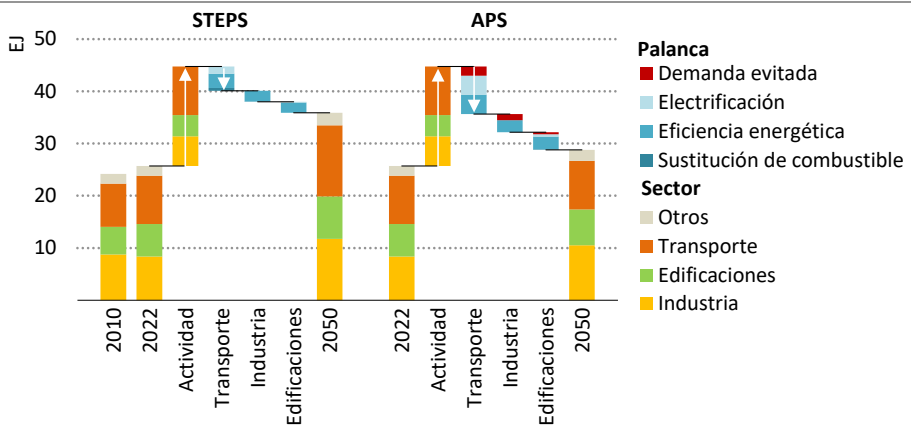
Figura 1 ▶ Consumo de energía final por escenario en ALC
