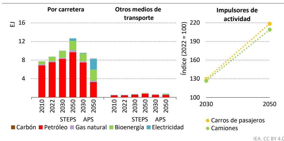
Figura 3 ▶ Consumo de combustible en el transporte por tipo y escenario en ALC
