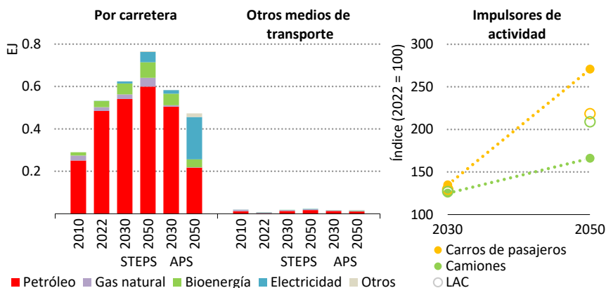
Figura 3 ▶ Consumo de combustibles en el transporte por tipo y escenario en Colombia
