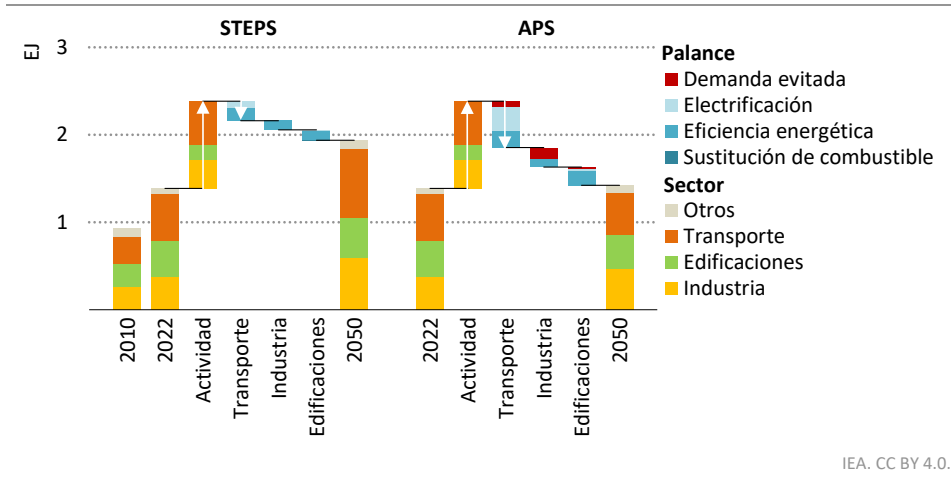
Figura 1 ▾ Consumo de energía final por escenario en Colombia
