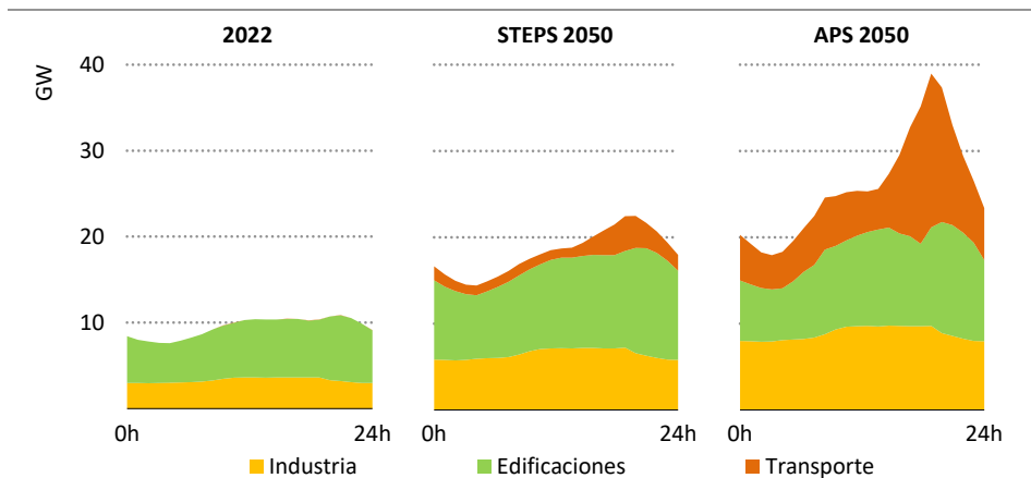
Figura 5 ▶ Perfil de carga eléctrica promedio diaria por escenario en Colombia
