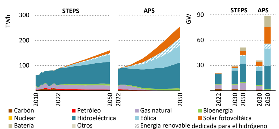
Figura 6 ▶ Generación y capacidad de electricidad por combustible y escenario en Colombia
