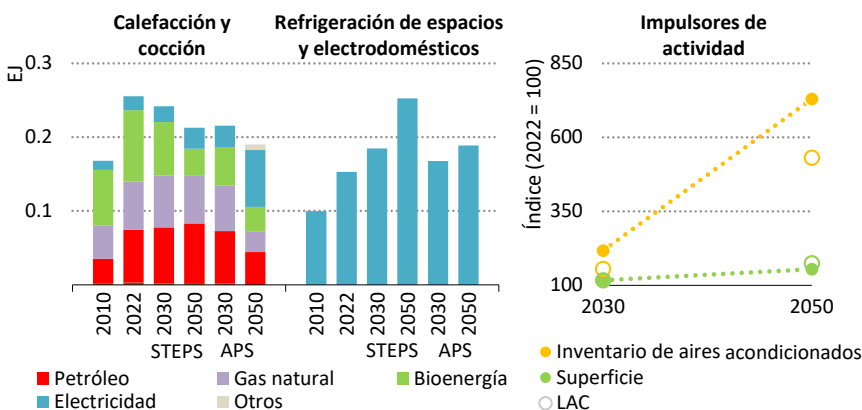
Figura 4 ▶ Consumo de combustible en edificaciones por tipo y escenario en Colombia
