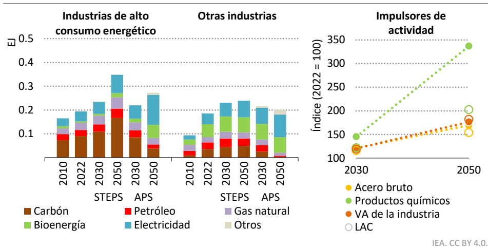
Figura 2 ▾ Consumo de combustible en la industria por tipo y escenario en Colombia
