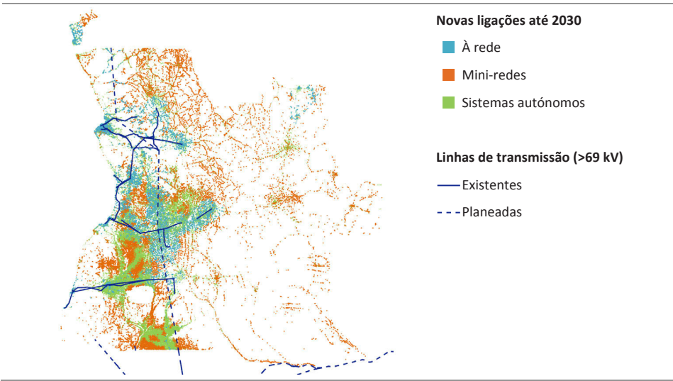
Figura 6.2C ▶ Soluções de acesso à eletricidade em Angola por tipo no Caso Africano
