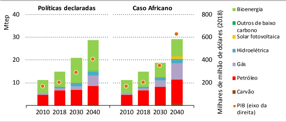
Figura 6.2A ▶ Demanda de energia primária e PIB em Angola
