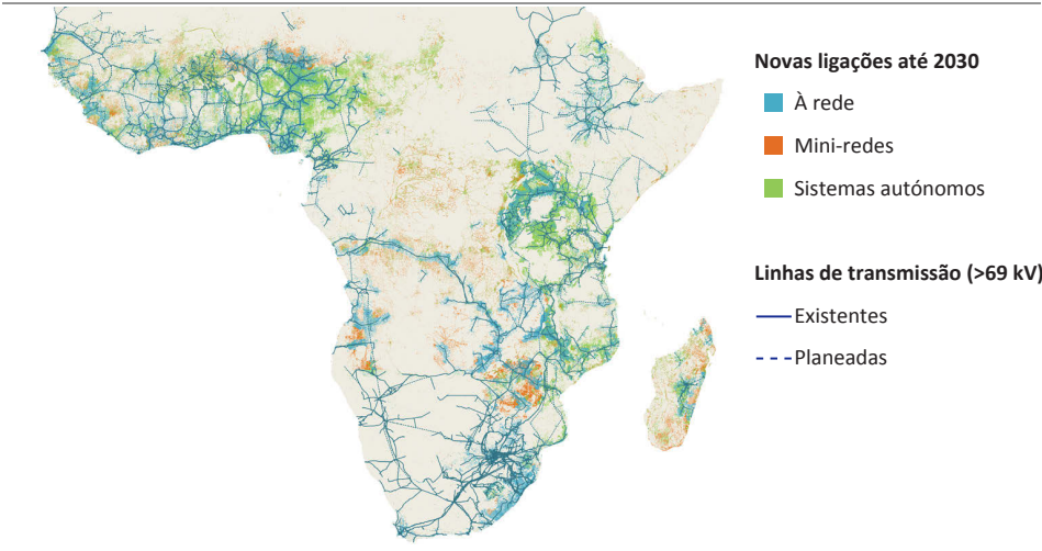
Figura 6.1C ▶ Soluções de acesso à eletricidade na África subsariana por tipo no Caso Africano
