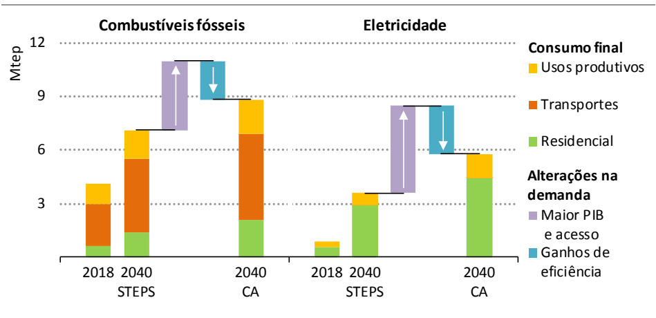
Figura 6.2D ▶ Consumo final de energia em Angola
