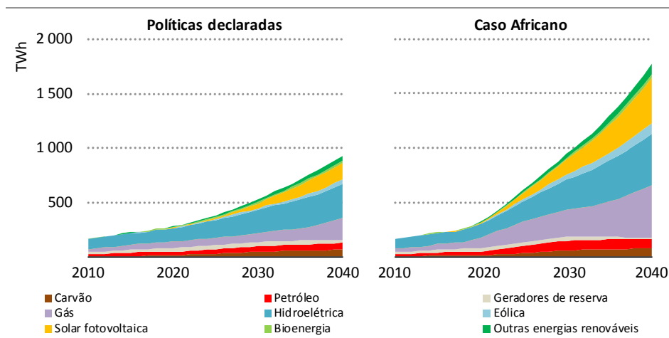
Figura 6.1B ▶ Produção de eletricidade por via tecnológica na África subsariana
