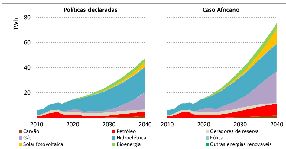
Figura 6.2B ► Produção de eletricidade por via tecnológica em Angola
