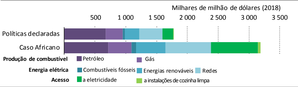
Figura 6.1G ▶ Necessidades cumulativas de investimento na África subsariana, 2019-2040
