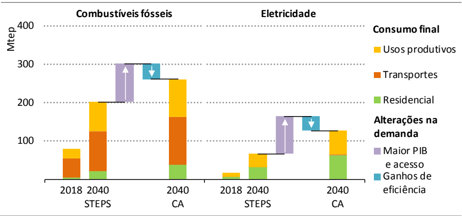
Figura 6.1D ▶ Consumo energético final na África subsariana
