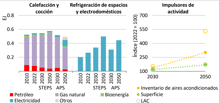
Figura 4 ▶ Consumo de combustible en edificaciones por tipo y escenario en Argentina
