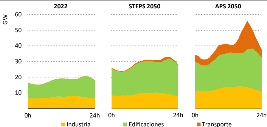
Figura 5 ▷ Perfil de carga eléctrica promedio diaria por escenario Argentina
