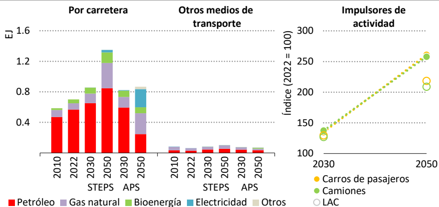
Figura 3 ▶ Consumo de combustible en el transporte por tipo y escenario en Argentina
