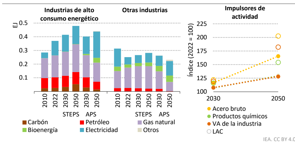
Figura 2 ▾ Consumo de combustible en la industria por tipo y escenario en Argentina
