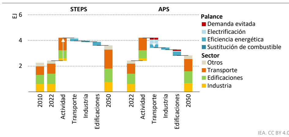
Figura 1 ▾ Consumo de energía final por escenario en Argentina
